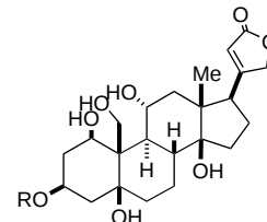
1a R = L-rhamnose 1b R = H
